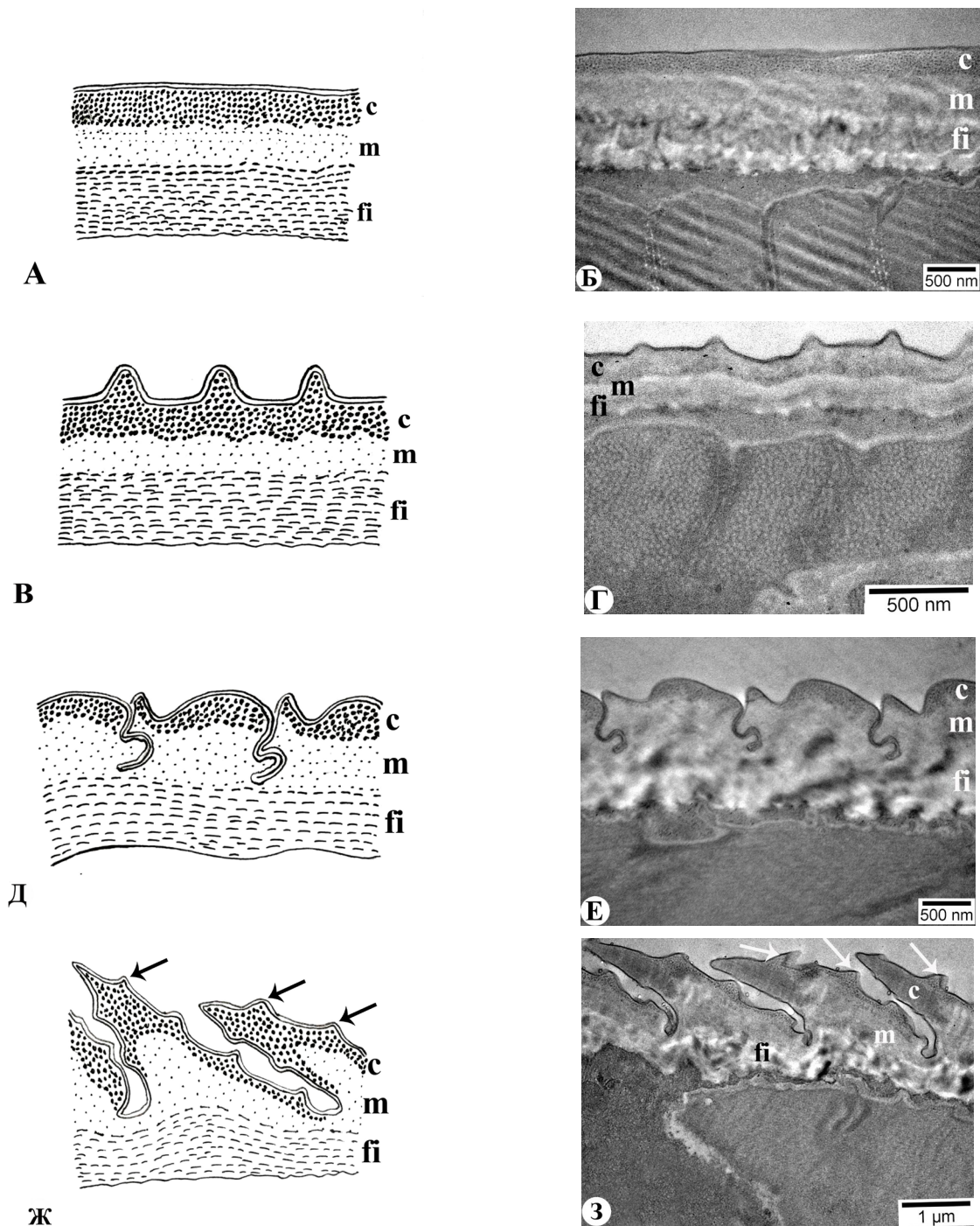
Рис. 2. Ультраструктура кутикулы и латеральных крыльев нематоды T. tenuis . А, В, Д, Ж – схематические рисунки; Б, Г, Е, 3 – электронограммы; А, Б – форма кутикулы без латеральных крыльев; В, Г – крылья в форме «ребня»; Д, Е – крылья в форме «крючков»; Ж, 3 – крылья в форме «шипа»; c – кортикальный слой; m – гомогенный или средний слой; fi – фибриллярный или волокнистый слой. Объяснения даны в тексте
